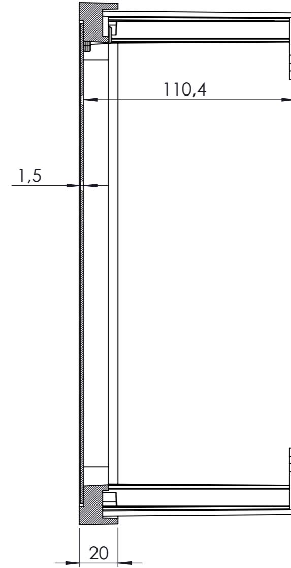
KESIT A-A
