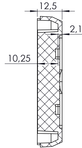
KESİT A-A
