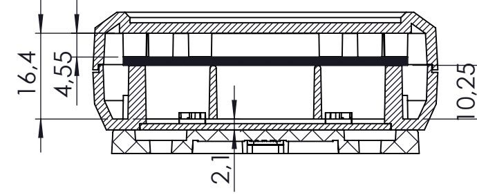
KESİT A-A ÖLÇEK 1 : 1
