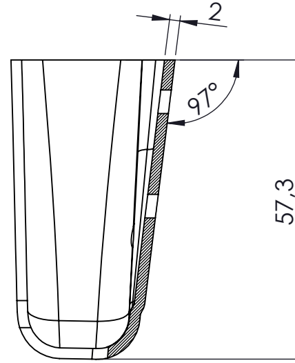
KESİT A-A
