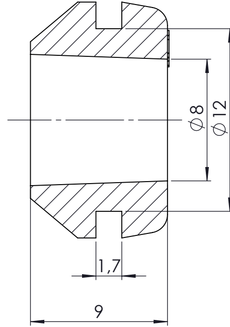
KESİT A-A
