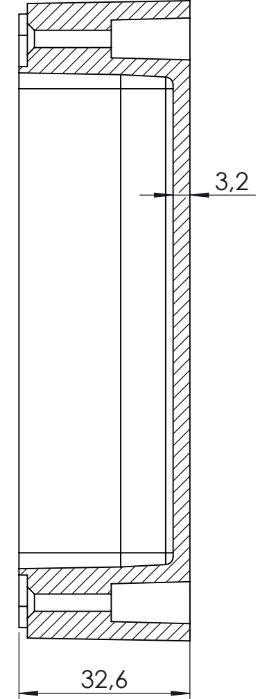
KESIT A-A
