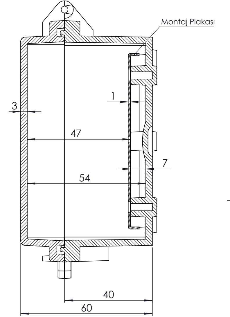
KESİT A-A
