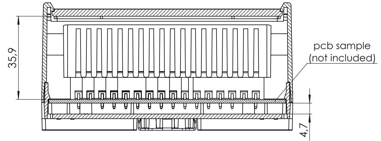
Section A-A
