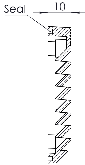
KESİT A-A
