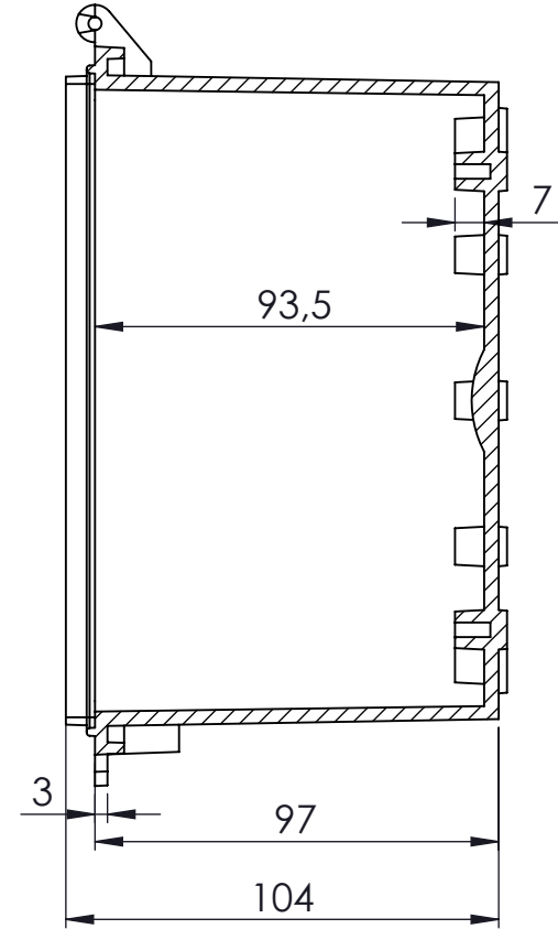
KESIT A-A
