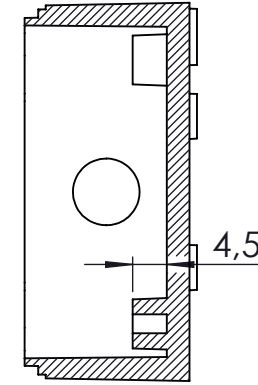
KESİT A-A
