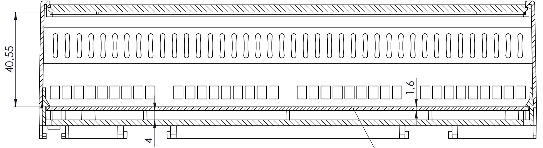
KESİT A-A
