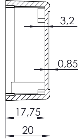
KESİT A-A
