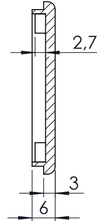
KESİT A-A
