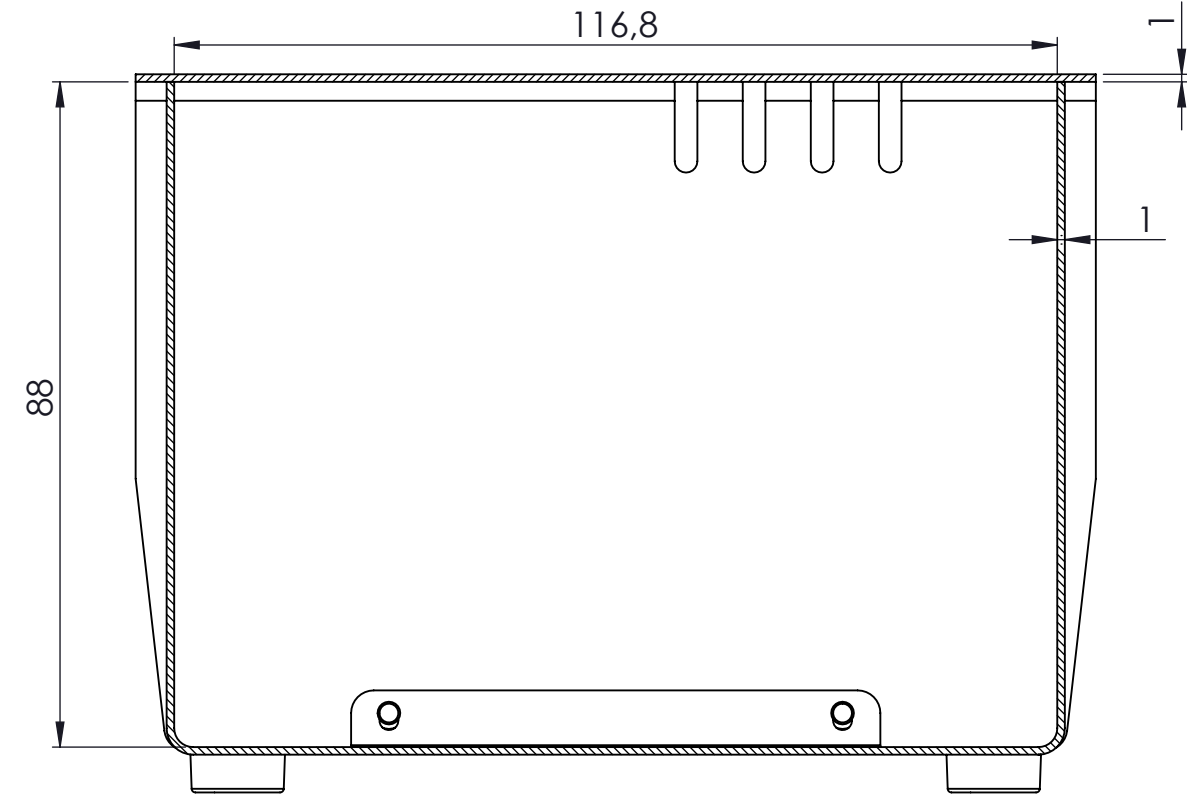
KESIT A-A
