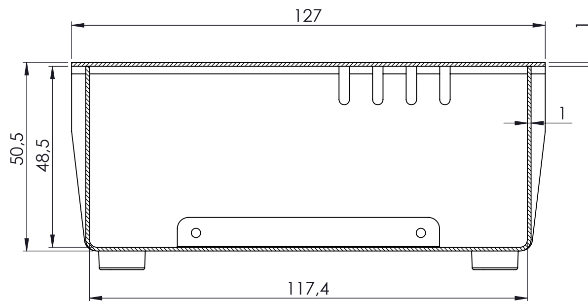
KESİT A-A
