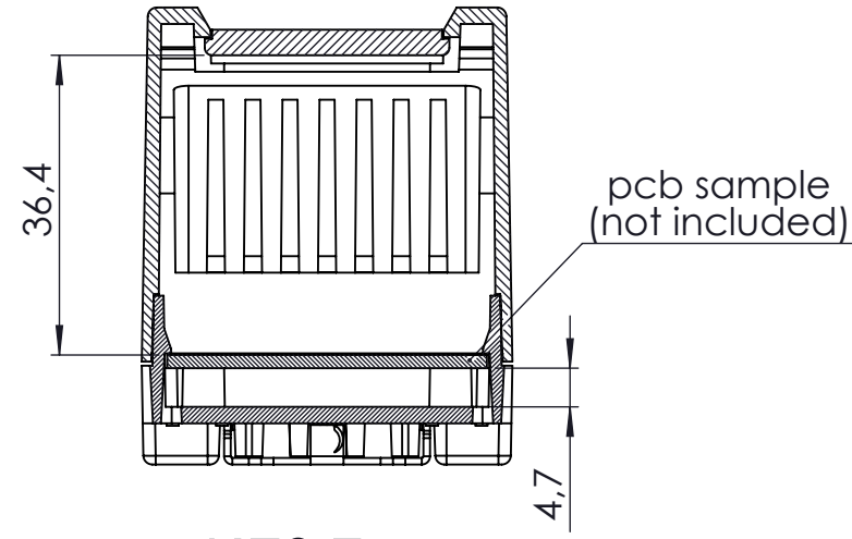
KESİT A-A
