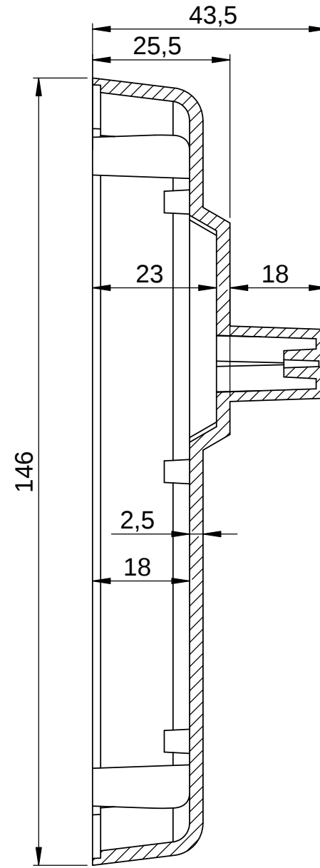
KESIT A-A
