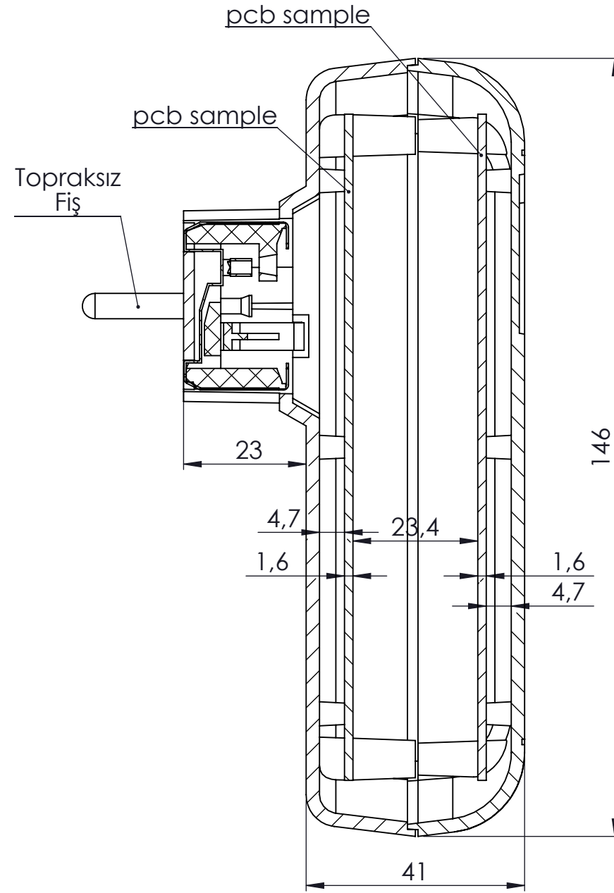
KESIT A-A
