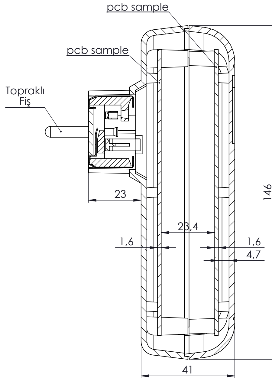
KESİT A-A
