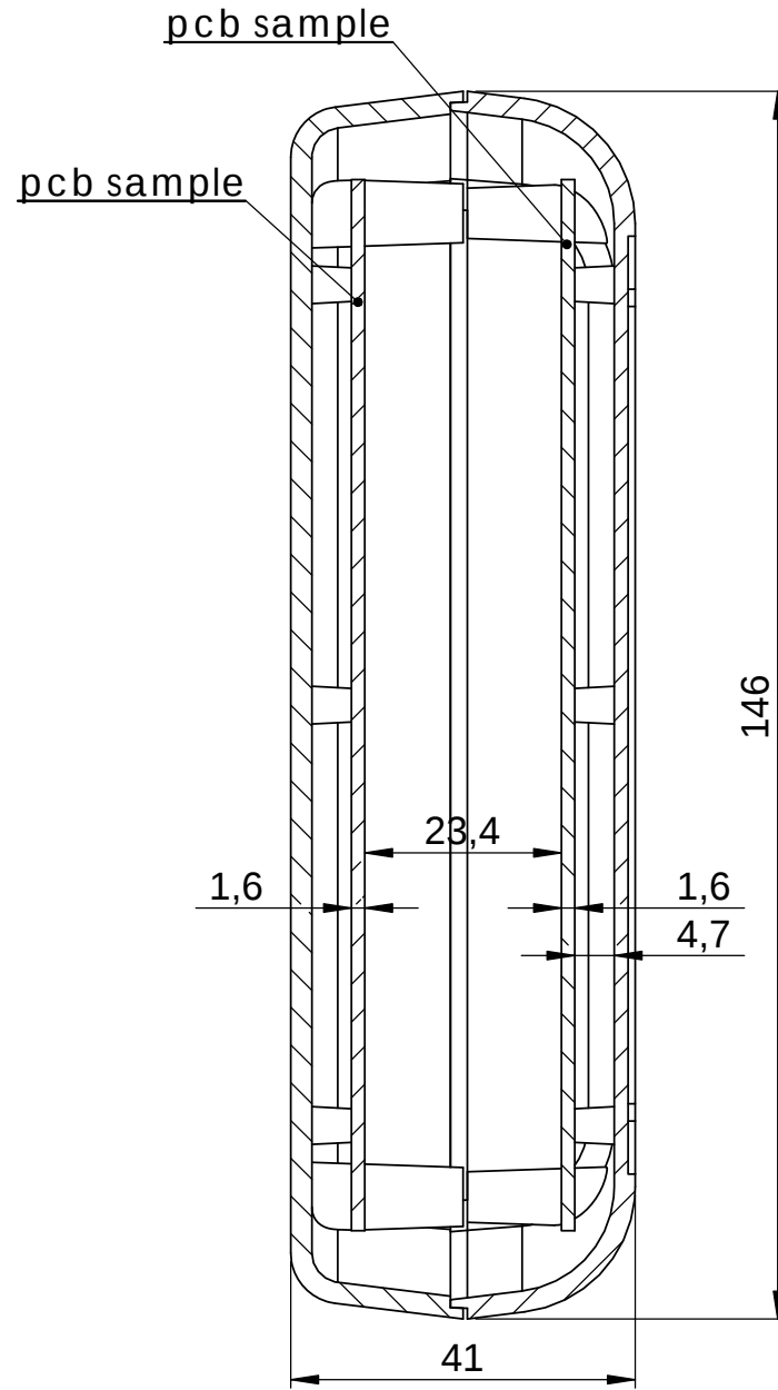
KESIT A-A
