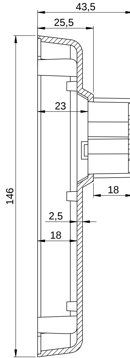
KESIT A-A
