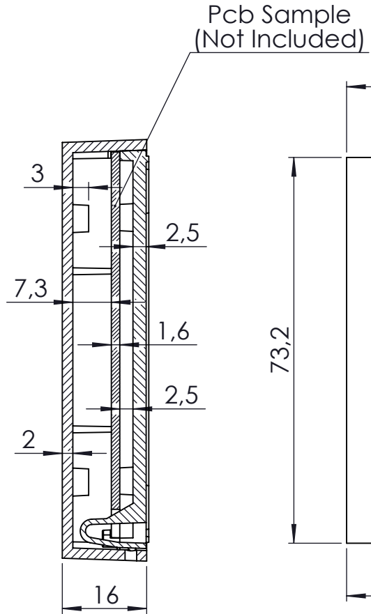
KESIT A-A
