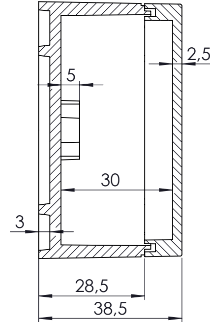
KESIT A-A
