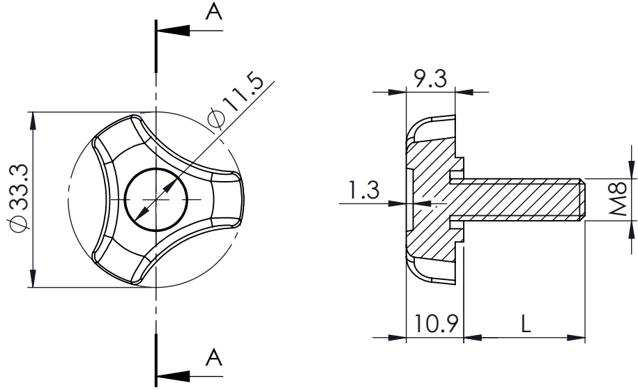
KESIT A-A
