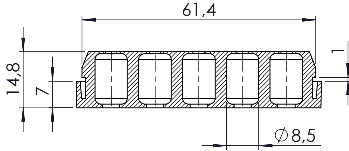
KESİT A-A
