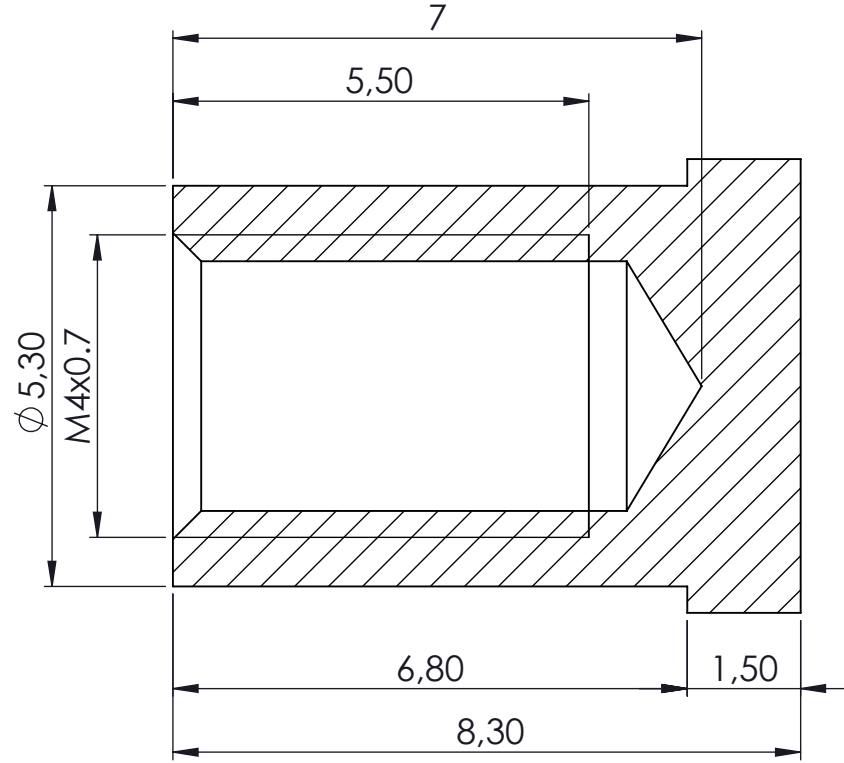
KESIT A-A
