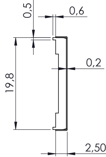
KESIT A-A
