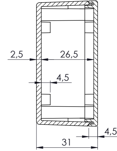
KESIT A-A
